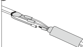
■ 슬리브 + 수축튜브 활용
