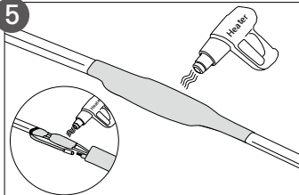
■ 도체/편조를 구분하여 마무리
